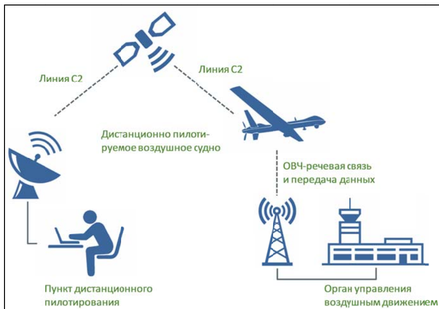
Рис. 12-2. Связь за пределами RLOS (BRLOS) через ретранслятор (как правило, через спутник)
