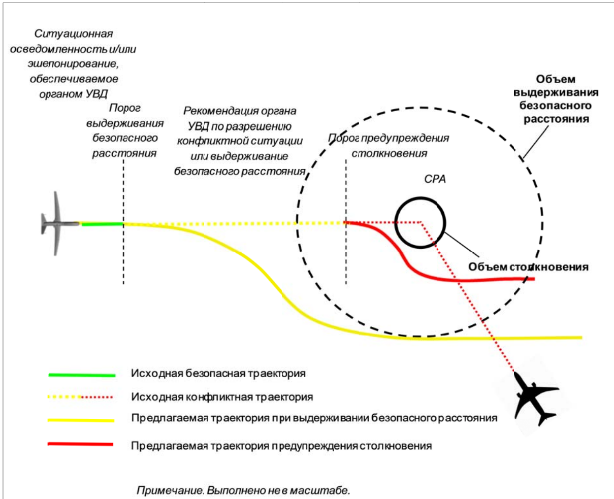
Рис. 10-3. Примеры разрешения конфликтных ситуаций в горизонтальной плоскости на основе RWC и PC
