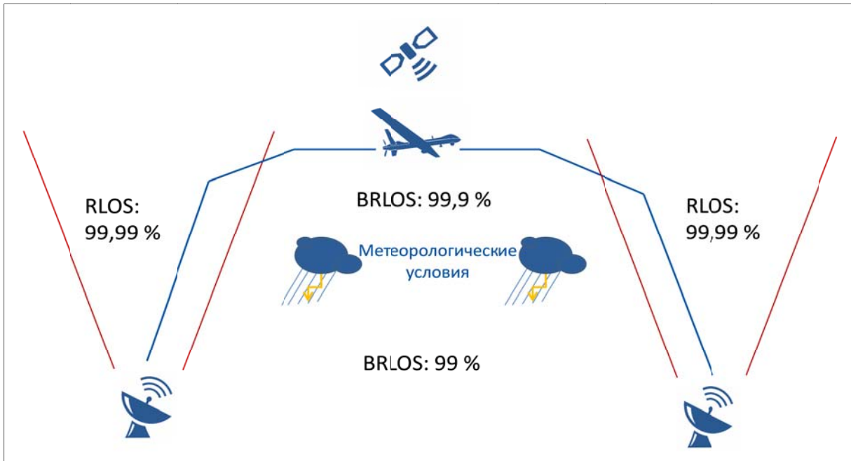
Рис. 11-3. Пример, иллюстрирующий готовность линии C2
