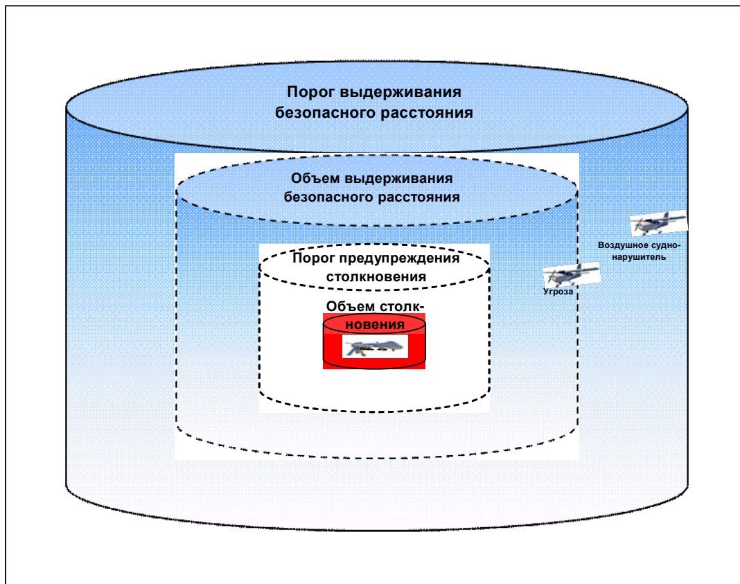
Рис. 10-2. Геометрия обеспечения RWC и ПС
